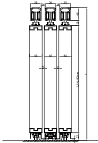
CASP-MW-3 Slide Door Max Door Width : 900 mm ₹ : 33,000/-*
