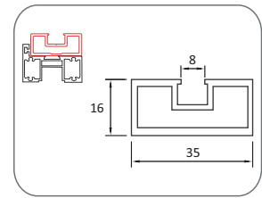
CASP-SP-3516 - DOOR FRAMED PROFILE
