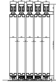
CASP-MW-5 Slide Door Max Door Width : 900 mm ₹ : 48,000/-*
