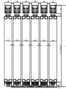
CASP-MW-6 Slide Door Max Door Width : 900 mm ₹ : 56,000/-*
